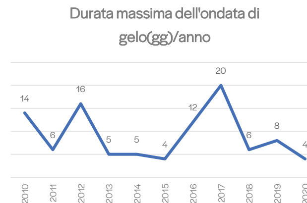
Figura 63: Andamento annuale della durata massima delle ondate di gelo dal 2010 al 2020. Fonte: elaborazione dati ARPAV
