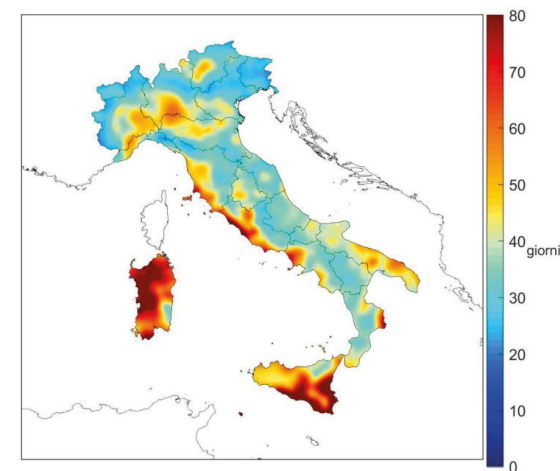
Figura 59: indice di siccità, giorni consecutivi- fonte ISPRA
