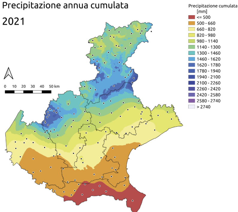
Figura 54: Precipitazioni in mm nel 2021 in Veneto
