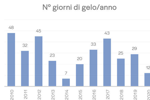
Figura 44: Andamento annuale del numero di giorni di gelo dal 2010 al 2020. Fonte: elaborazione personale con dati ARPAV
