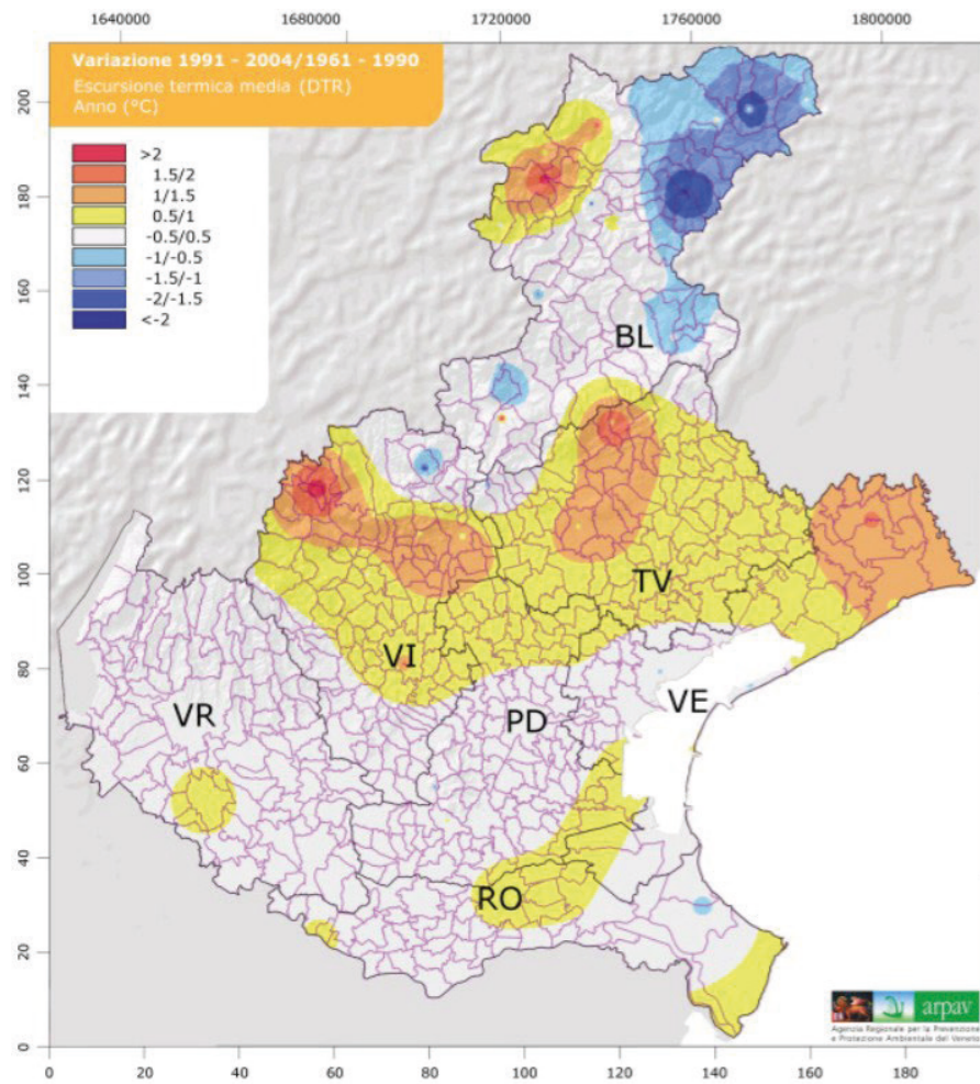
Figura 40: : Variazione 1961-1991 e 1992-2004 dell'escursione termica media annua in °C. Fonte: Atlante agro climatico del Veneto
