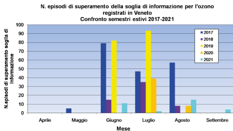
Figura 79: Distribuzione da aprile a settembre negli anni dal 2017 a 2021 delle concentrazioni di azoto_ fonte ARPAV
