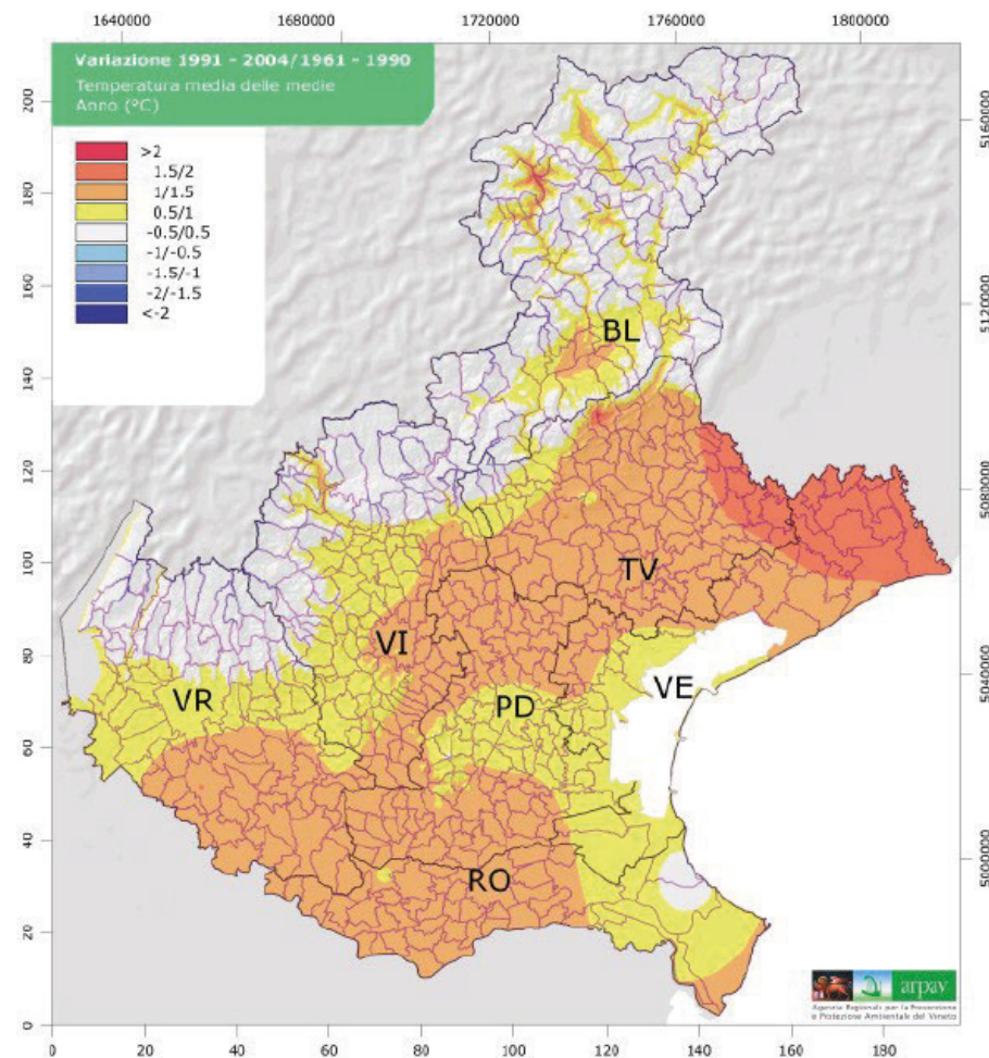
Figura 34: Variazione 1961-1991 e 1992-2004 delle temperature medie annuali in °C. Fonte: Atlante agroclimatico del Veneto -temperature ARPAV
