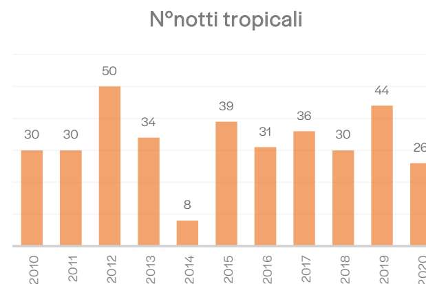
Figura 43: Andamento annuale del numero di notti tropicali dal 2010 al 2020. Fonte: elaborazione personale con dati ARPAV
