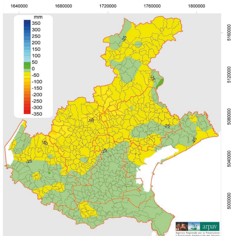
Figura 48: Inverno: precipitazioni medie stagionali in mm. Fonte: Atlante climatico del Veneto – Precipitazioni, ARPAV
