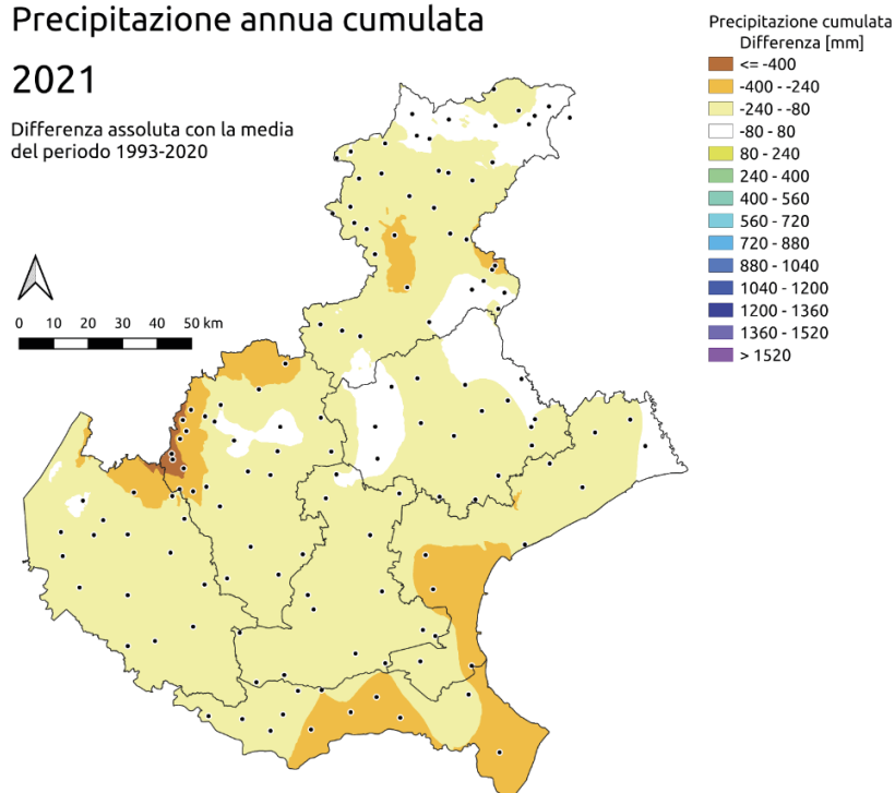
Figura 55: differenza assoluta con media del periodo 1993-2020
