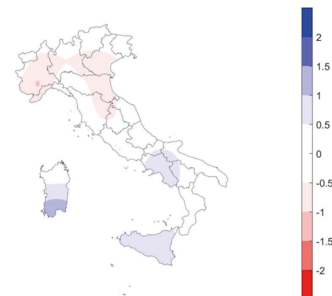
Figura 58: indice di siccità SPI annuale 2021- fonte ISPRA
