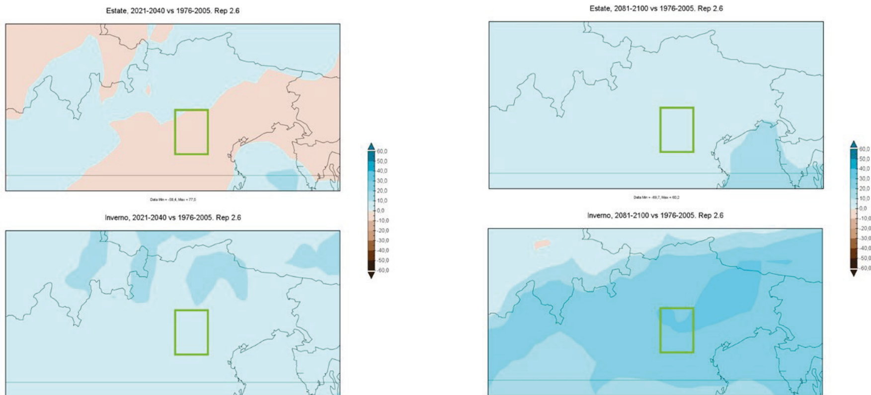
Figura 68: Variazione dell'anomalia delle precipitazioni in pianura padana durante la stagione invernale ed estiva per lo scenario RCP 2.6 per l'intervallo temporale 2021-2040 (a sinistra) e per l'intervallo 2081-2100 (a destra) rispetto al riferimento 1976-2005.
