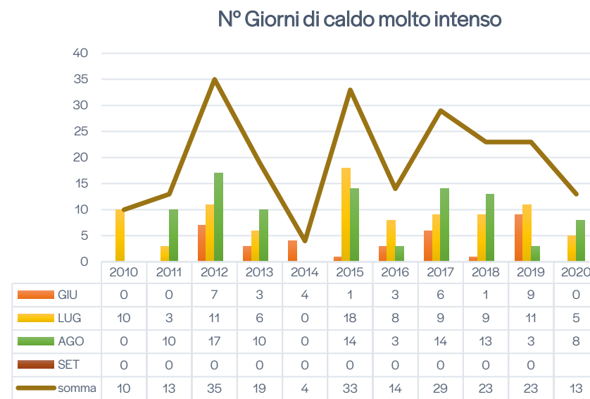
Figura 45: Andamento delle giornate di caldo molto intenso nel periodo 2010-2020. Fonte: elaborazione dati ARPAV
