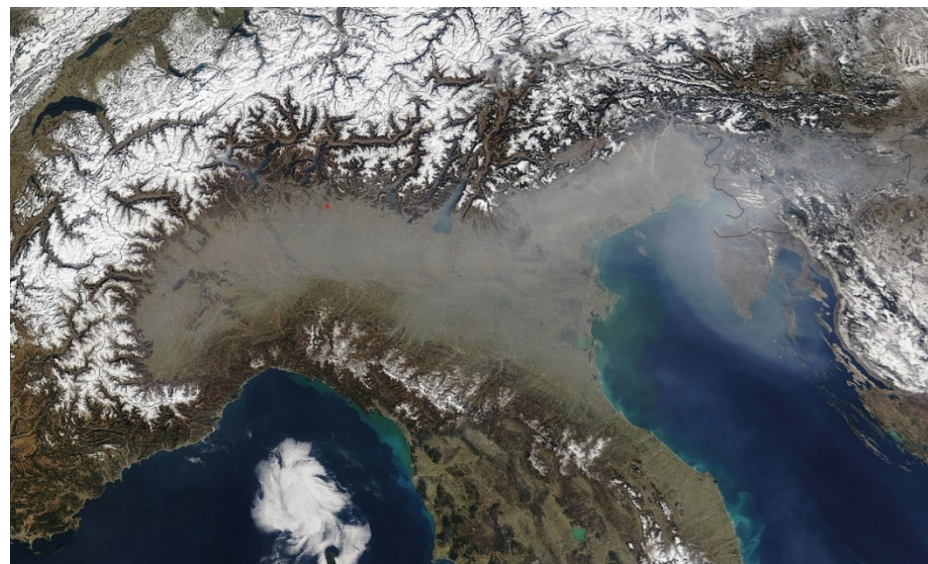
Figura 75: immagine satellitare invernale della Pianura Padana e delle aree limitrofe. Fonte NASA-MODIS
