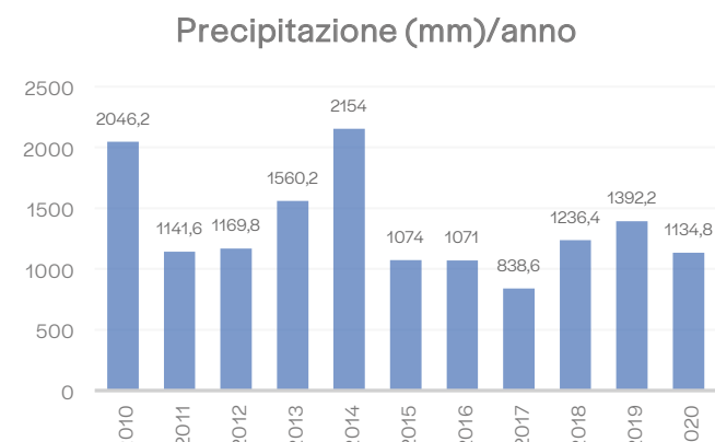
Figura 56: Andamento delle precipitazioni annuali, in mm di pioggia caduta, periodo 2010-2020. Fonte: elaborazione personale con dati ARPAV
