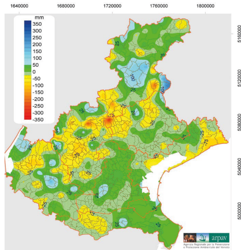
Figura 47: Variazione 1981-2010 e 1961-1990 delle precipitazioni medie annue in mm. Fonte: Atlante climatico del Veneto – Precipitazioni, ARPAV.
