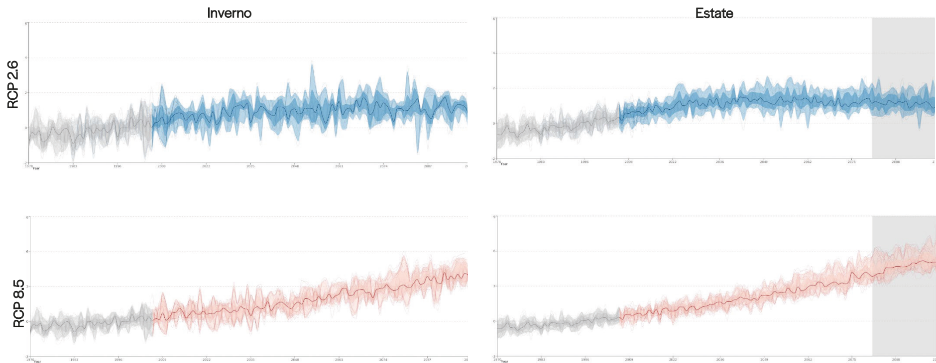
Figura 64: Andamento medio dell'anomalia delle temperature invernali ed estive nella regione mediterranea fino al 2100 rispetto al periodo 1976-2005 per gli scenari RCP 2.6 (in blu), e 8.5 (in rosso). Fonte: IPCC WGI Interactive Atlas
