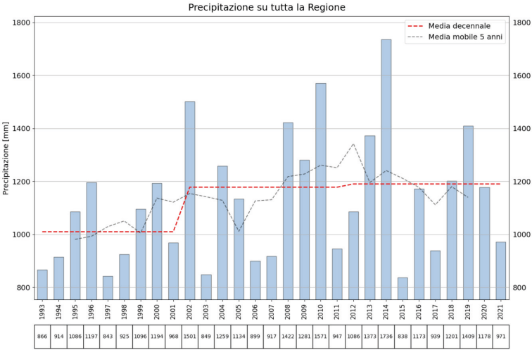
Figura 52: Precipitazioni annuali nel periodo 1993-2021
