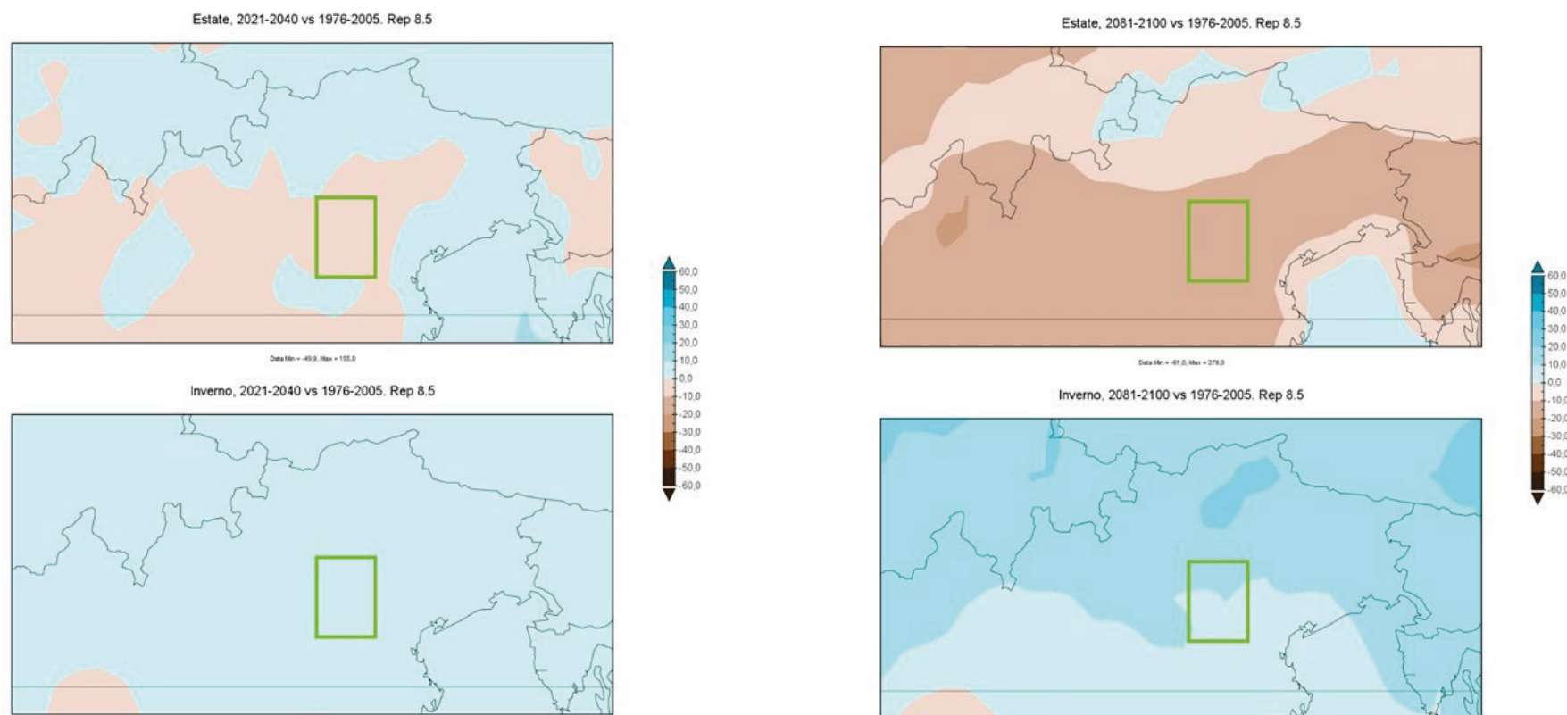
Figura 69: Variazione dell'anomalia delle precipitazioni in pianura padana durante la stagione invernale ed estiva per lo scenario RCP 8.5 per l'intervallo temporale 2021-2040 (a sinistra) e 2081-2100 (a destra) rispetto al riferimento 1976-2005. Fonte: IPCC WGI.
