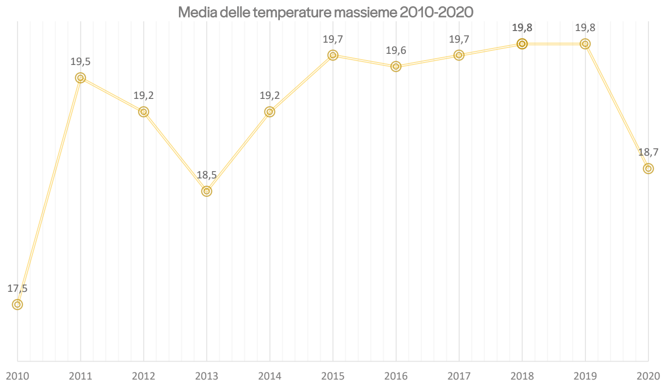
Figura 42: Andamento delle medie delle temperature massime nel periodo 2010-2020. Fonte: elaborazione dati ARPAV
