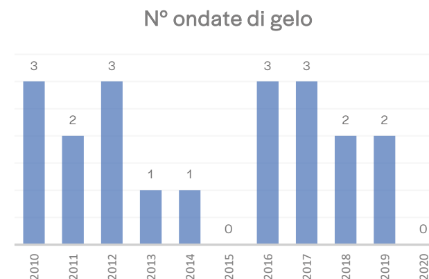
Figura 62: Andamento annuale del numero delle ondate di gelo dal 2010 al 2020. Fonte: elaborazione personale con dati ARPAV.
