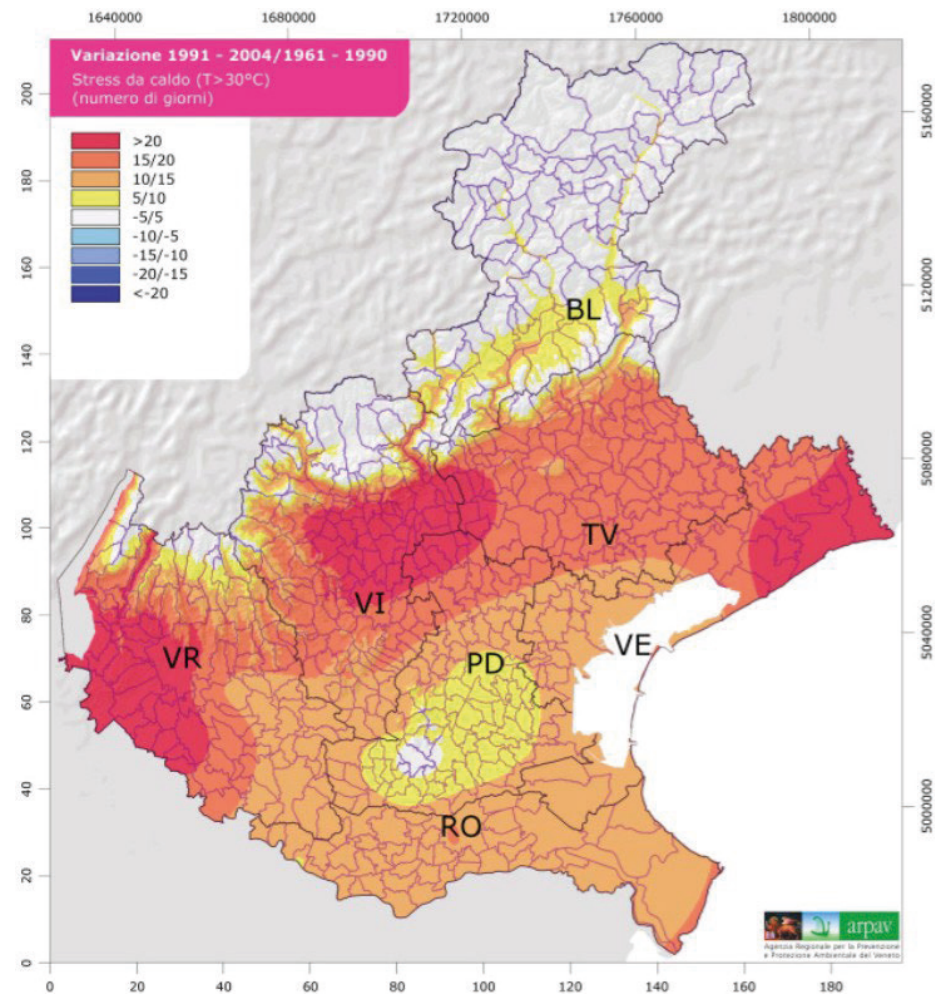
Figura 41: Variazione 1961-1991 e 1992-2004 dell'indice stressa da caldo annuo in n°giorni. Fonte: Atlante agroclimatico del Veneto
