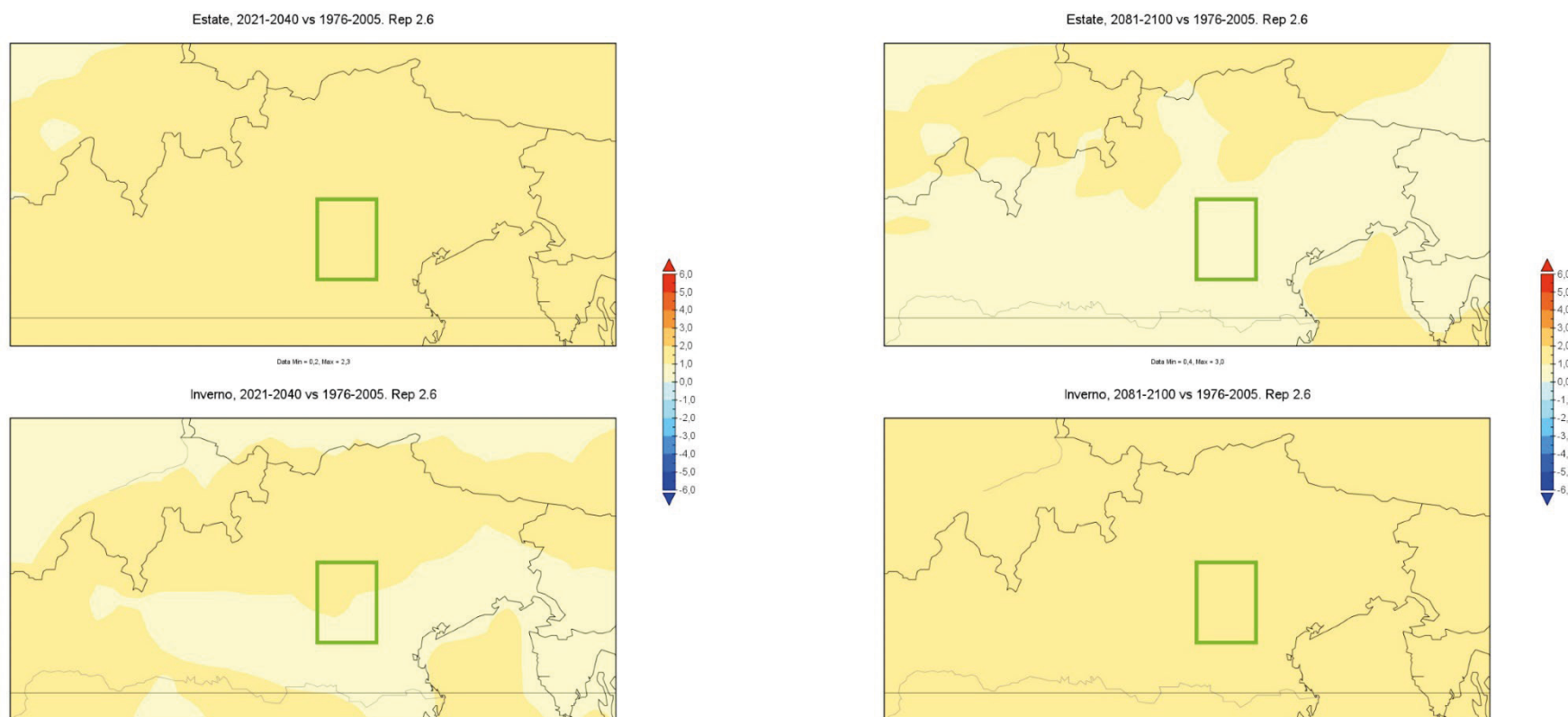
Figura 65: Variazione dell'anomalia di temperatura della pianura padana durante la stagione invernale ed estiva per lo scenario RCP 2.6 per l'intervallo temporale 2021-2040 (a sinistra) e per l'intervallo 2081-2100 (a destra) rispetto al riferimento 1976-2005. Fonte: IPCC WGI Interactive Atlas, elaborazione su applicazione Panoply. Il riquadro in verde localizza la provincia di Vicenza.
