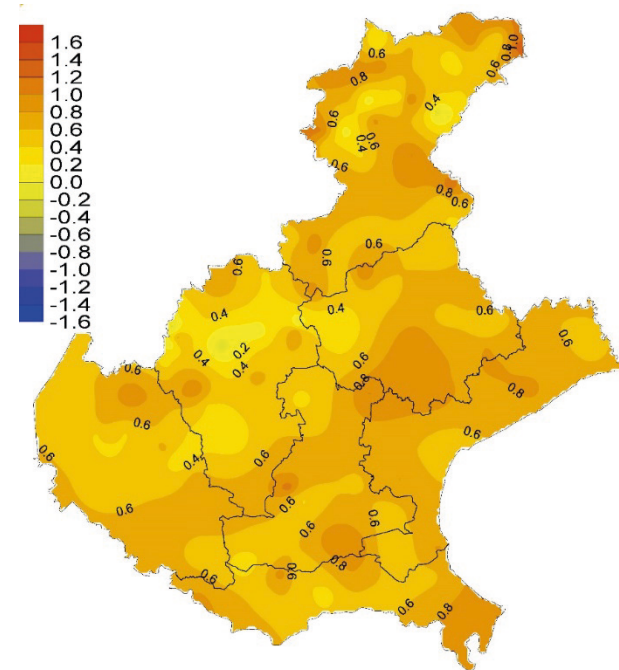
Figura 39: temperatura massima 2020 rispetto alla media 1994 - 2019. Fonte: ARPAV
